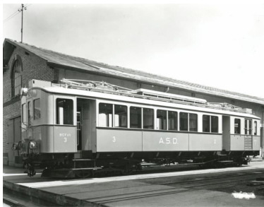
ASD BCFe 4/4 no 3 (Set no 7)
