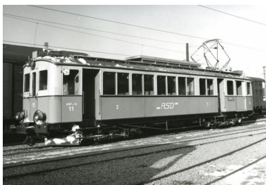
ASD ABFe 4/4 no 11 (Set no 10)
